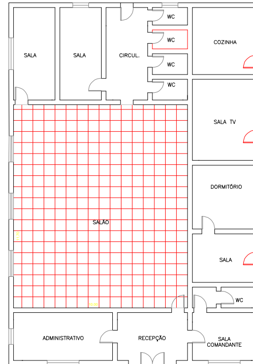
PLANTA-BAIXA A CONSTRUIR ESC. 1/100
