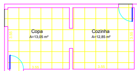
PLANTA-BAIXA A DEMOLIR ESC. 1/100
