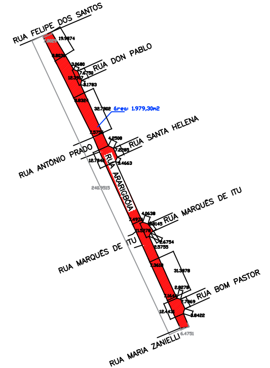
LEVANTAMENTO PLANIMÉTRICO RUA ARARIGBOIA – VILA FESTI
