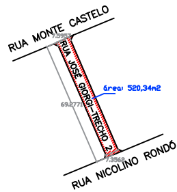
LEVANTAMENTO PLANIMÉTRICO RUA JOSÉ GIORGI – VILA FESTI – TRECHOS 1 E 2
